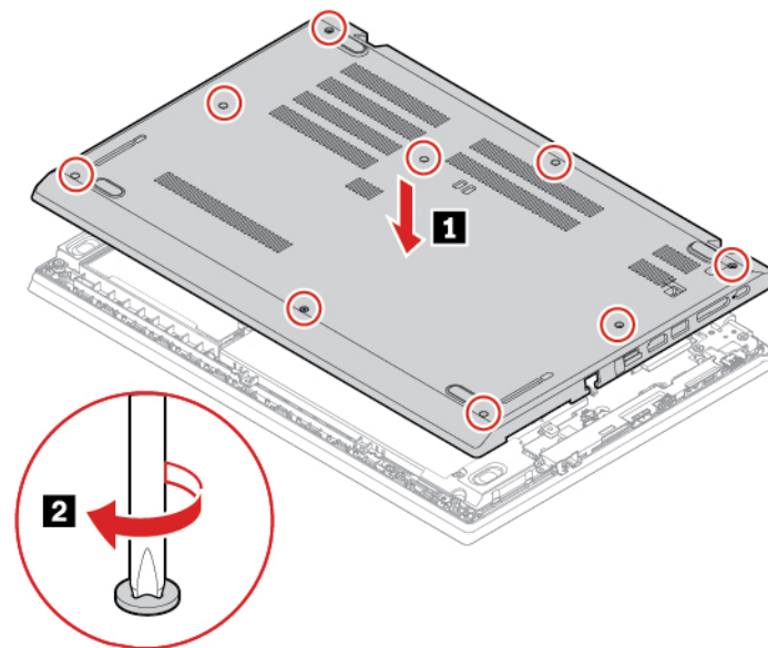
Figure 7. Installation du cache de la base pour le L590
