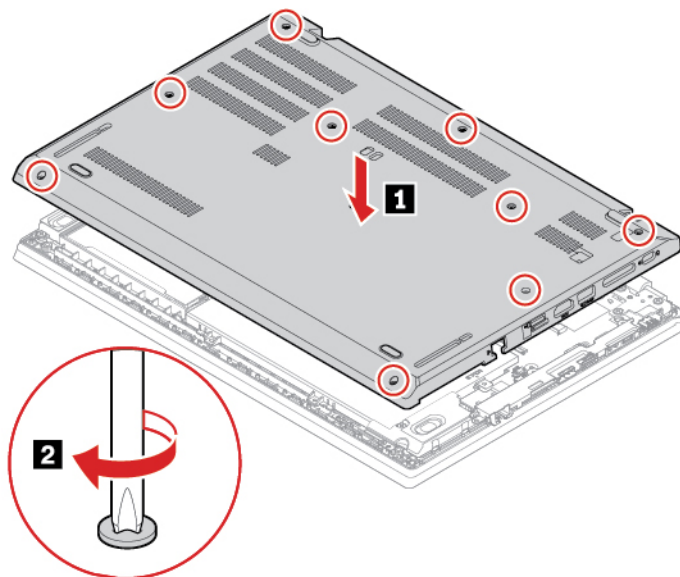
Figure 6. Installation du cache de la base pour L490
