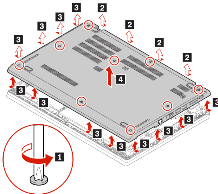
Figure 5. Retrait du cache de la base pour le L590
